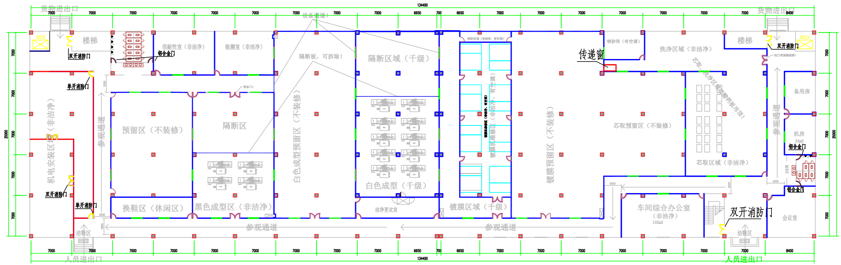
1F 车间平面规划图 1:100
