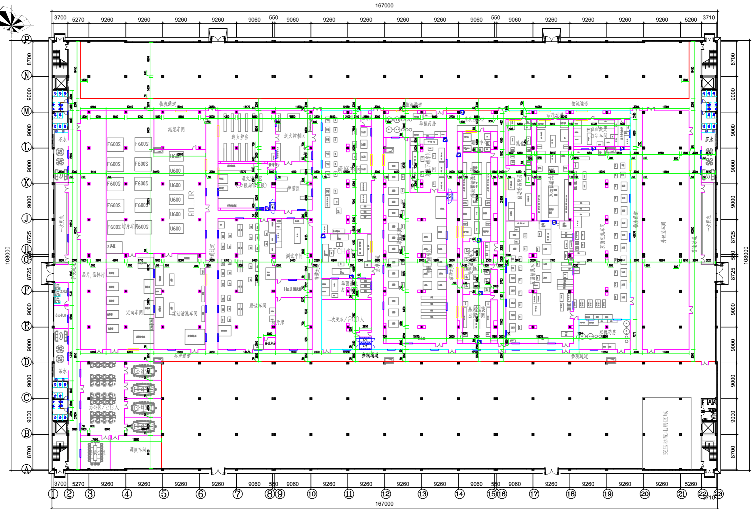
1F 结构平面图
