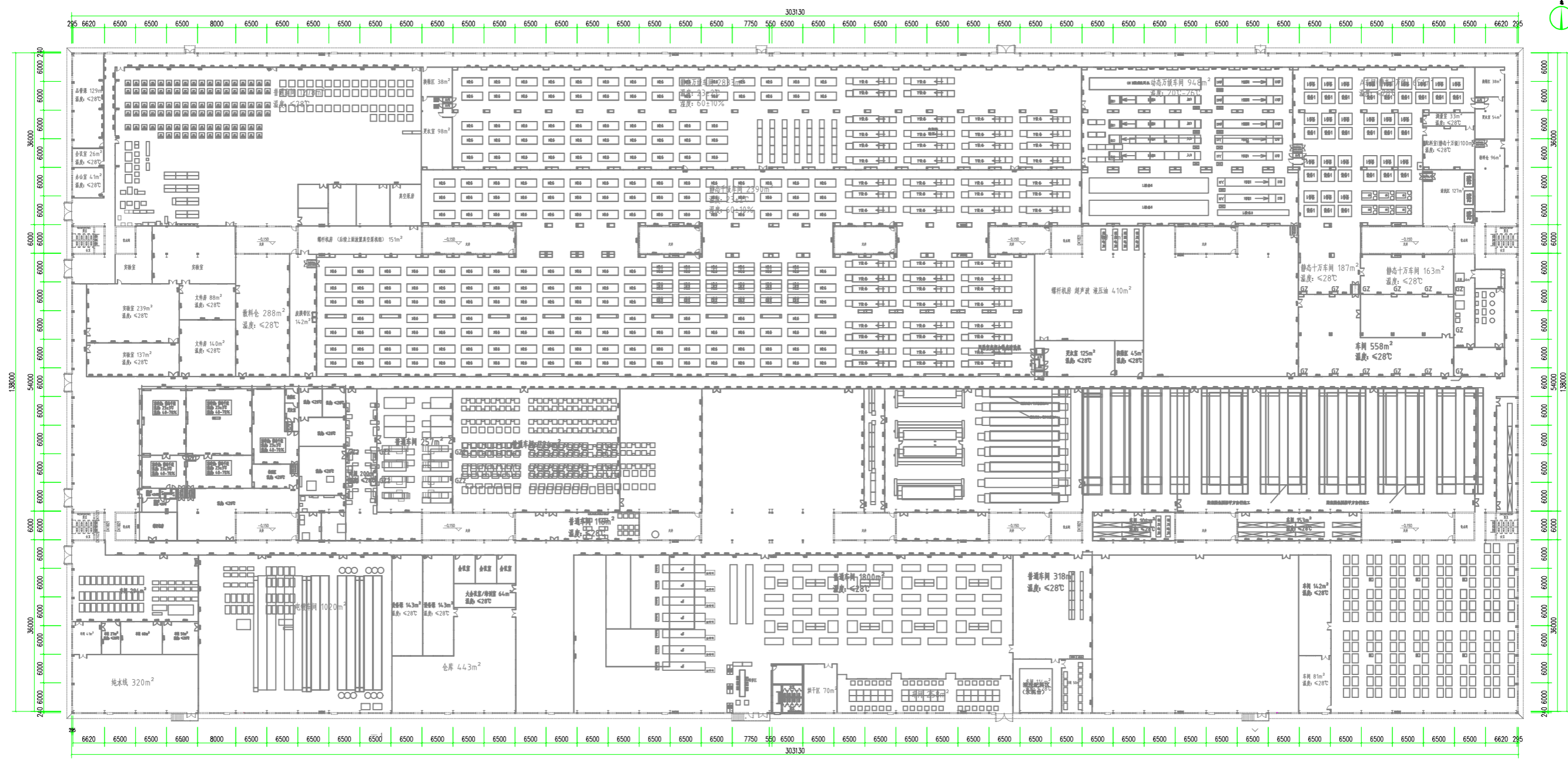
电器件场地平面规划 1:500
