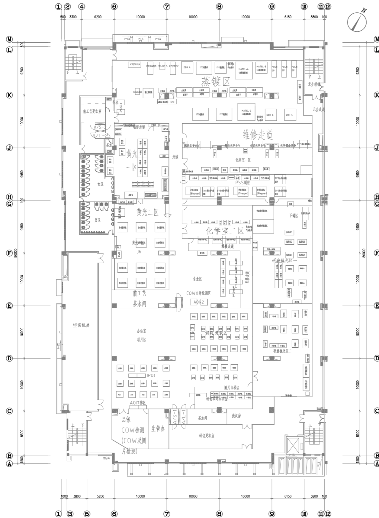
A1芯片厂平面规划图 1:150
